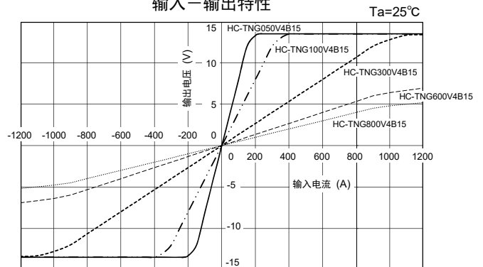
输入—输出特性
