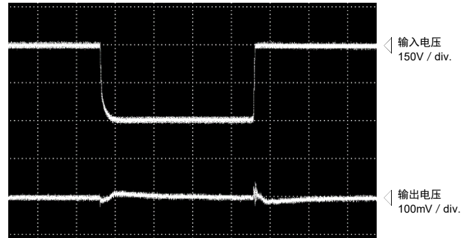
干扰特性(dv/dt影响)
